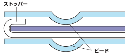
ストッパータイプ断面
