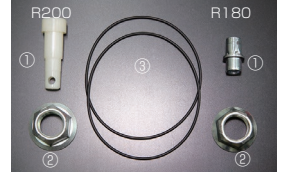
R200/R180 デフパーツ R200 R180 ①プリーザー ¥320 ¥310 ②ピニオンロックナット ¥1,510 ¥360 ③リテーナーOリングSET — ¥540 (2025.10.30 更新)
