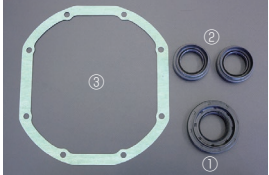
R200 デフパーツ (2025.4.9 更新) ①ピニオンオイルシール ¥980 ②サイドオイルシール ¥430/1ヶ ③デフカバーパッキン ¥2,440
