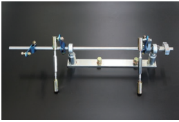
2TG ロッド式リンケージキット
