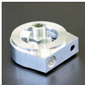
オイルブロック 品番: NTS 適応: A型, U20, CA, 4AG 価格 ¥10,700
