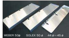
●L型 アルミヒートプレート (組み込みタイプ) SOLEX, WEBER, OER 40φ~45φ 本体 ¥5,500 ●L型 アルミヒートプレート (くり下げタイプ) SOLEX 44, 50φ WEBER 50φ 本体 ¥7,000 ※金具付き 本体 ¥6,000
