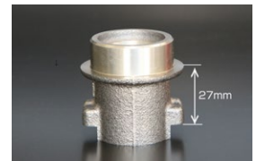
A12 クラッチスリーブ(27mm) ¥1,900 ■適合 A12標準品 A14A15にクロモリ軽量フライホイールを装着した時に交換必要。
