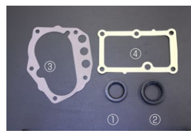
71C, 71B パッキン&シール ①フロントオイルシール ¥280 ②リアオイルシール ¥430 ③フロントカバーパッキン ¥990 ④71Cシフトハウジングパッキン (R32タイプ¥470 シルビア¥830)
